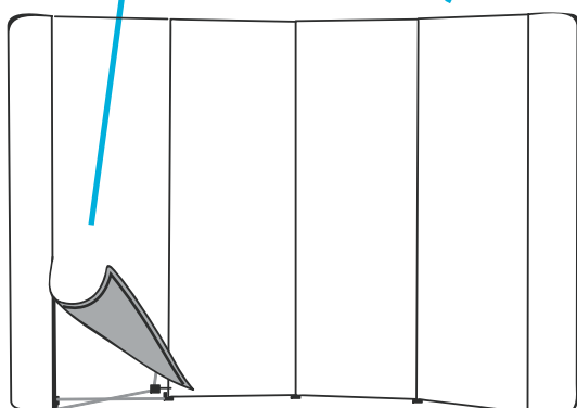
Velikost sestavy Pop Up 4x3 - PU01 š. 3000 x hl. 300 x v. 2300 mm
